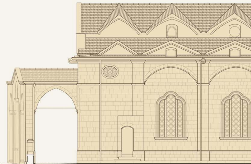
Νότια όψη (σχέδιο Ι&Α Φιλίππου, Paolo Vitti)
